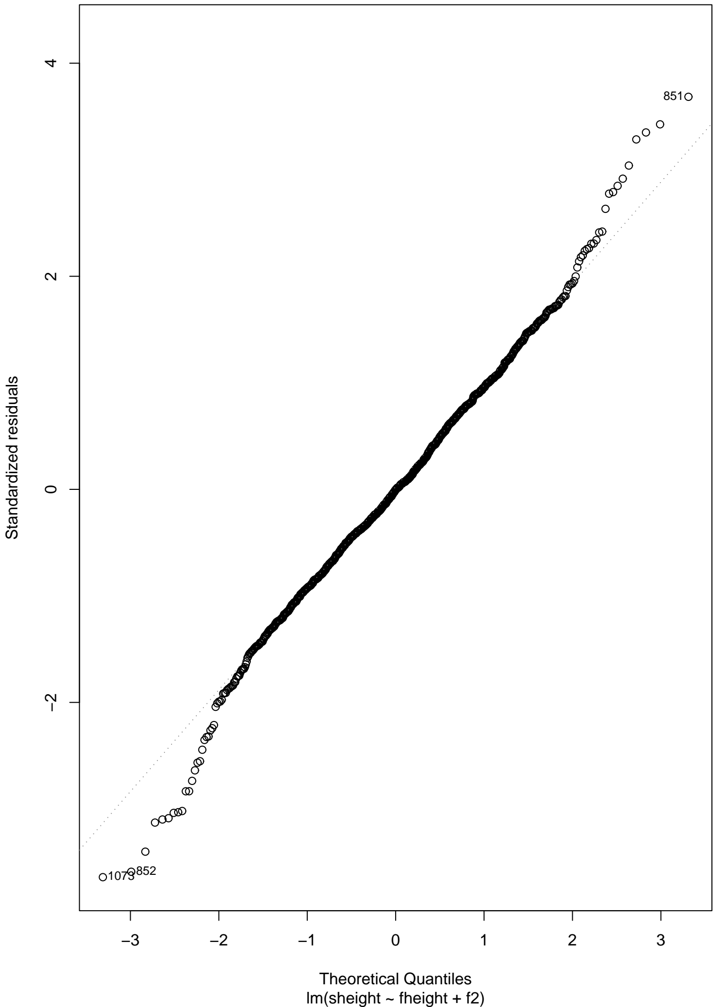
Normal Q-Q
